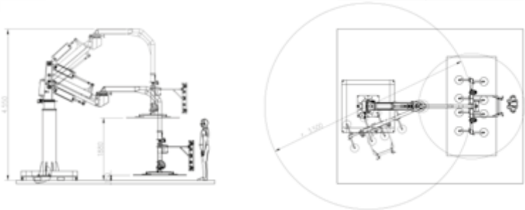
MANIPOLATORE CON BRACCIO A PANTOGRAFO PER ASSERVIMENTO CENTRI DI LAVORO. MANIPULATOR WITH PANTOGRAPH ARM FOR WORK CENTRES TENDING.
